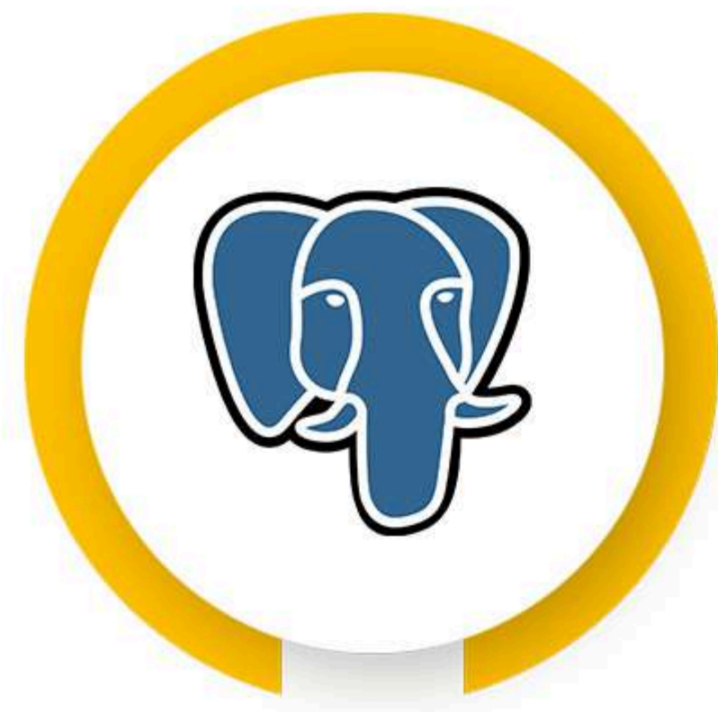
POSTGRESQL
