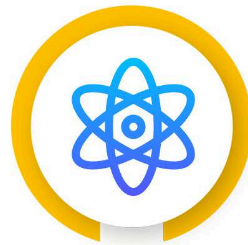
REACT.JS
