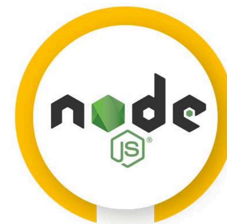
NODE.JS
