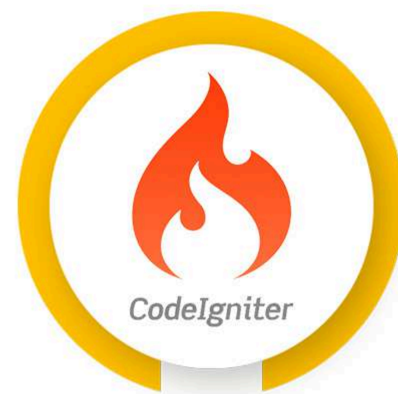
CODEIGNITER
