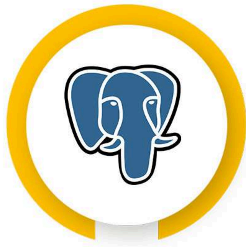
POSTGRES SQL
