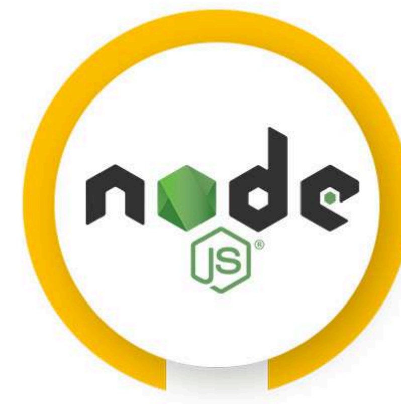
NODE.JS
