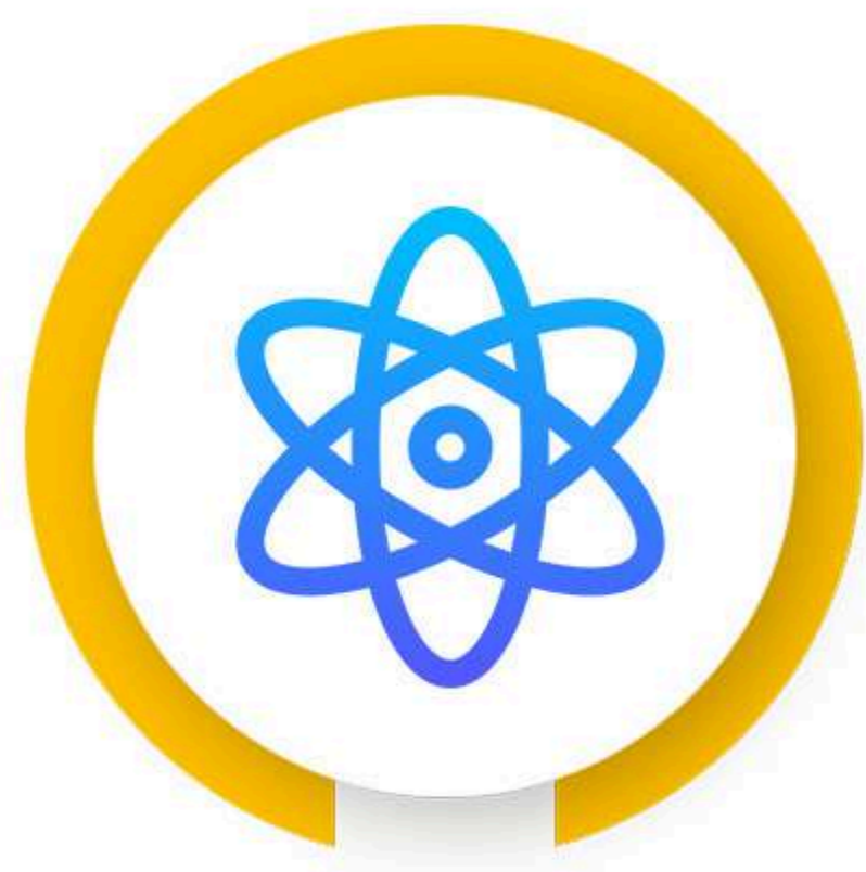
REACT.JS
