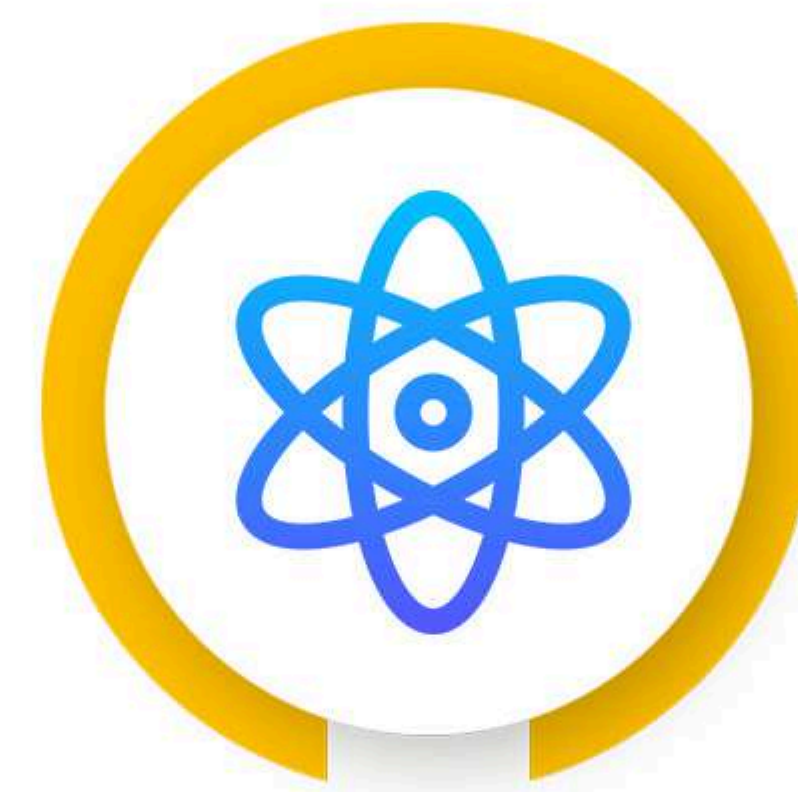
REACT.JS
