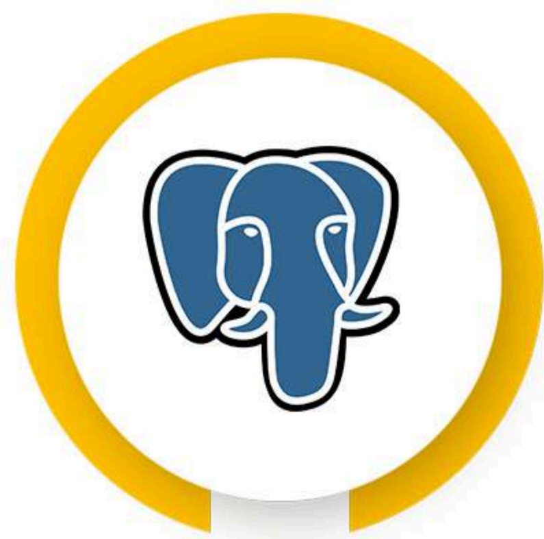
POSTGRES SQL
