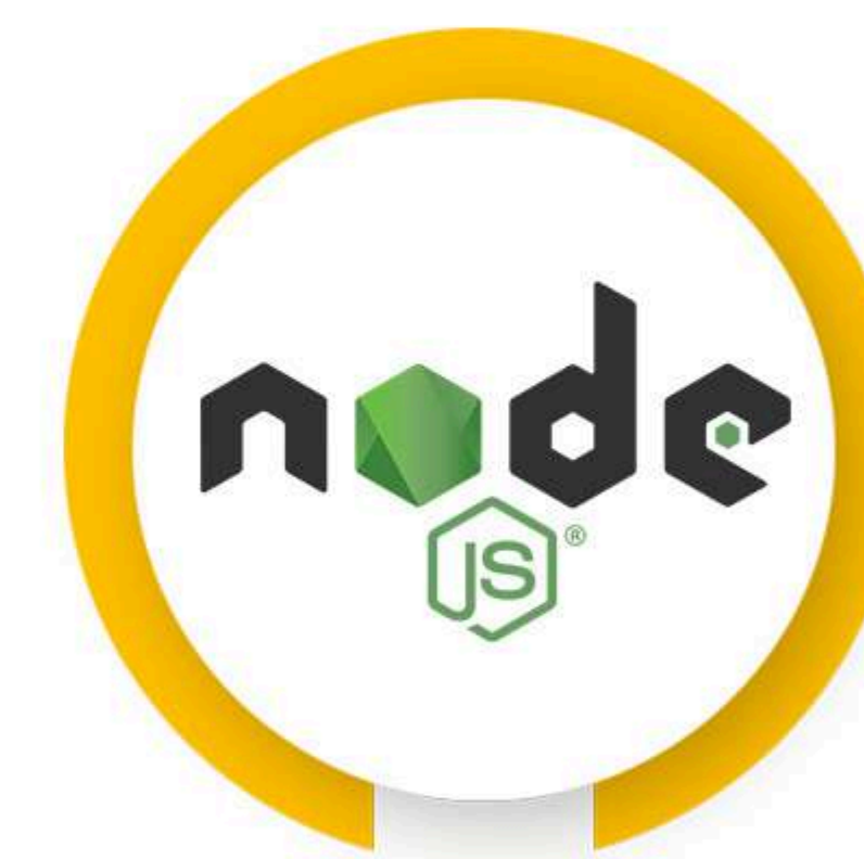
NODE.JS
